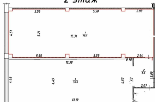
2 этаж
